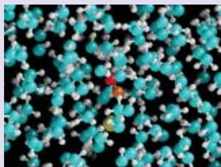
シアン化ナトリウム水溶液中におけるシアン化物イオンの振動状態緩和 (左) 水溶液のスナップショット (右) イオンの伸縮振動に関する波動関数の時間変化 t = 0 psにおいて第一励起状態にあったイオンが、まわりの水分子にエネルギーを受け渡しながら約 100 ps かけて基底状態へと緩和している。
