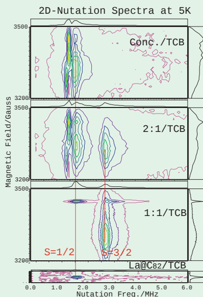
図2 2次元ニューテーション法でみた電子スピンの様子
