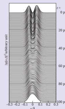
シアン化ナトリウム水溶液中におけるシアン化物イオンの振動状態緩和 (左) 水溶液のスナップショット (右) イオンの伸縮振動に関する波動関数の時間変化 t = 0 psにおいて第一励起状態にあったイオンが、まわりの水分子にエネルギーを受け渡しながら約 100 ps かけて基底状態へと緩和している。
