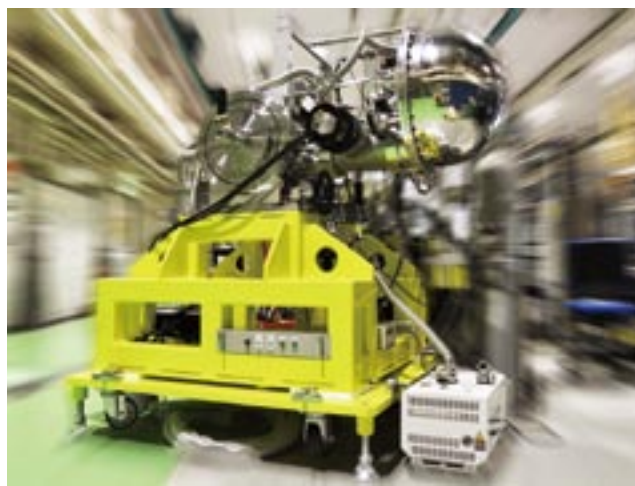
新ビームライン BL6U 用に開発された角度分解電子分光装置
