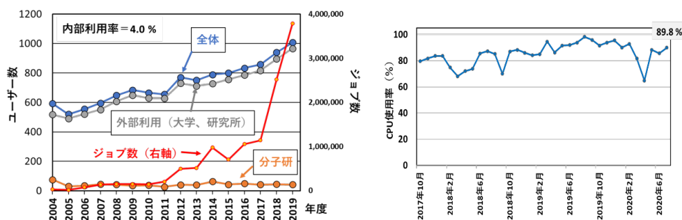
図Ⅳ-1: 計算科学研究センターの利用ユーザー数・ジョブ数 (左) と CPU 使用率 (右)
