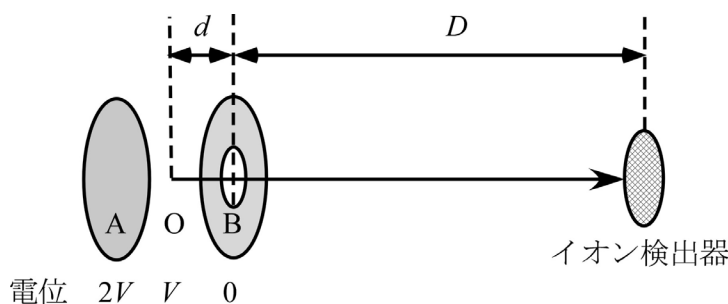
【図5】TOF 質量分析器（1段加速）
