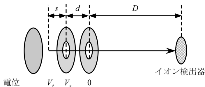
【図6】TOF 質量分析器（2段加速）
