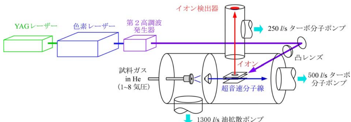
【図8】実験装置の模式図
